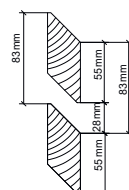
45° abgeschrägt/ 45° biseauté
