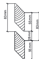
45° abgeschrägt/ 45° biseauté
