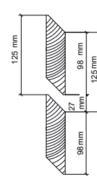
mit Zwischenraum
