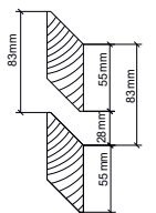
45° abgeschrägt/ 45° biseauté
