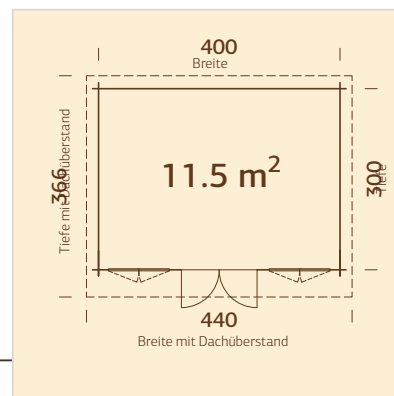
Grundriss
